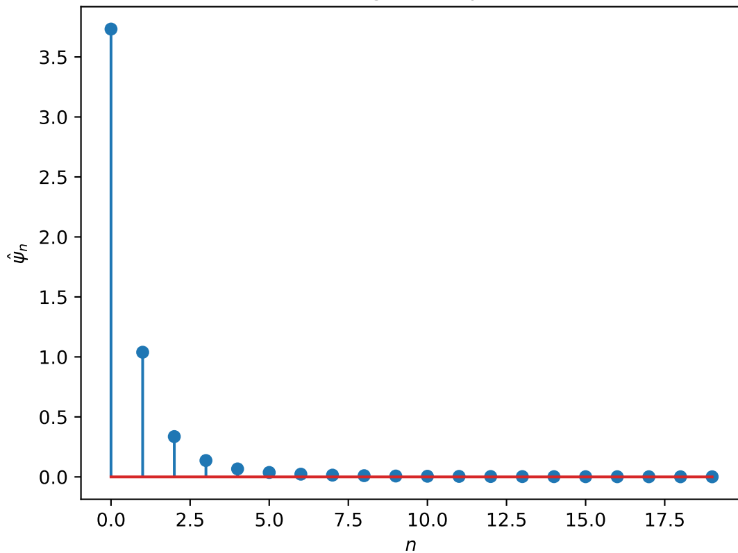
Fourier-Legendre Spectrum
